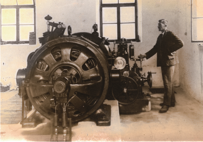
Blick in den Maschinenraum des E-Werks Gernmühle mit der als Erstausstattung eingesetzten Francis-Turbine (1920).
