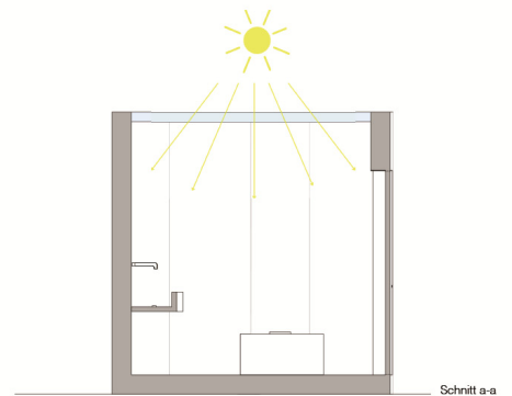
Schnitt a-a
