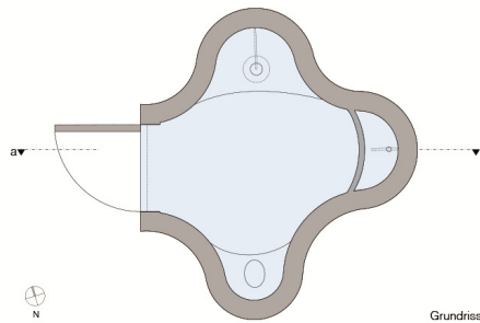
Grundriss
